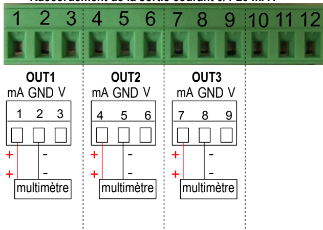
Raccordement de la sortie courant 0/4-20 mA :
