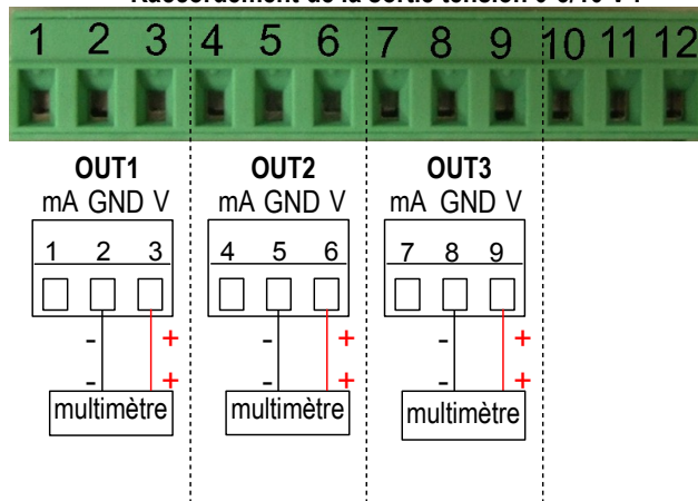
Raccordement de la sortie tension 0-5/10 V :
